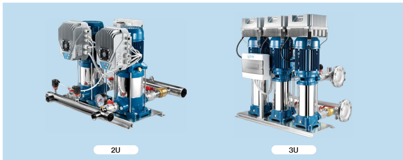
Grupos de presión de velocidad fija y velocidad variable con dos o tres bombas multicelulares
