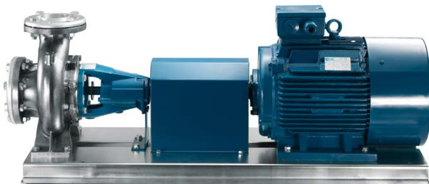
CAX-4CAX con motor contrabridas suministradas por separado
